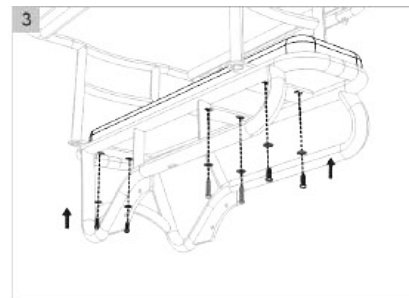
Hinteres Sitzkissen
